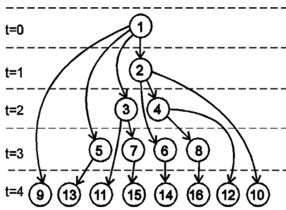
Рис. 1. Дерево потомков при послойном заполнении адресного пространства в условиях I_0=1 , \beta=1 .
